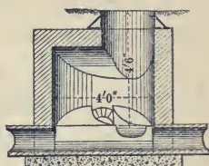
FIG. 3. SHALLOW MANHOLE.
